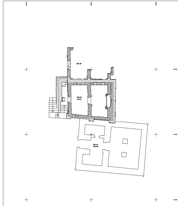
Tomb of Isidora, Palmyra, Syria Grabmal der Isidora, G. 127/28, Palmyra M. 1:100 Maßstab 1:100 Auf Grundlage der DTU-Cad-Datenbank Palmyra, G. 127/28, M. 1:100, 2008-2010 © 2013 CNR-IRPA
